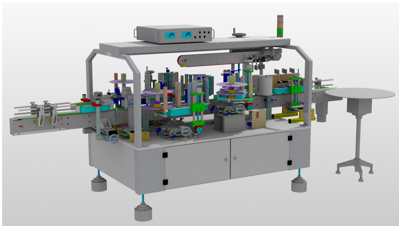
ALline C mit 3 ALritma-Etikettierköpfen
